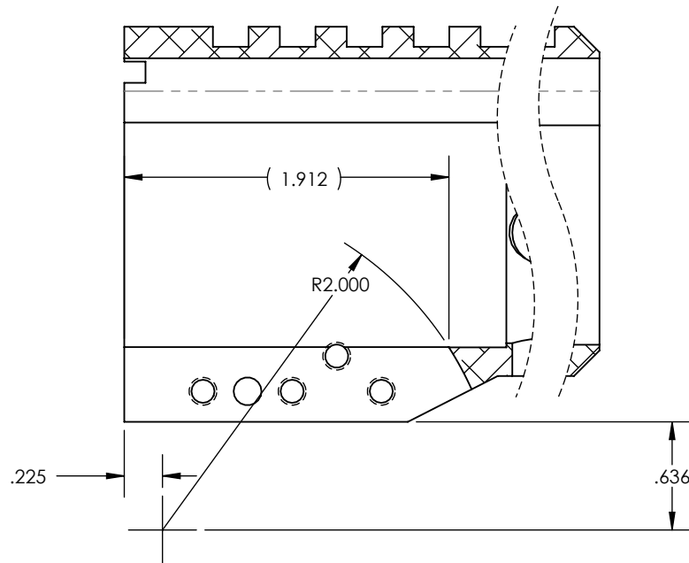
SECTION D-D
